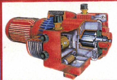
POMPES A VIDE, COMPRESSEURS GLS 962 - SERIE LFC 9000
